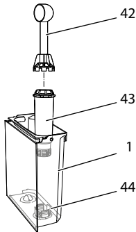
Abb. 24: Wasserfilter ein-/ausschrauben
