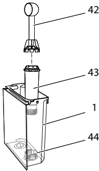
Fig. 24: Vissage/dévisage du filtre à eau
