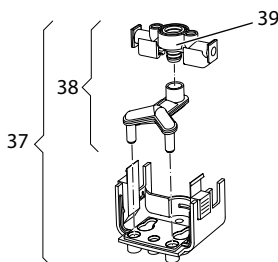
Abb. 23: Milcheinheit ausbauen
